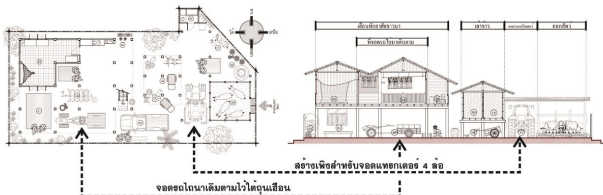
ภาพที่ 9 การจอดเครื่องจักรกลการเกษตรในผังเอื้อนชาวนาในกรณีศึกษา
