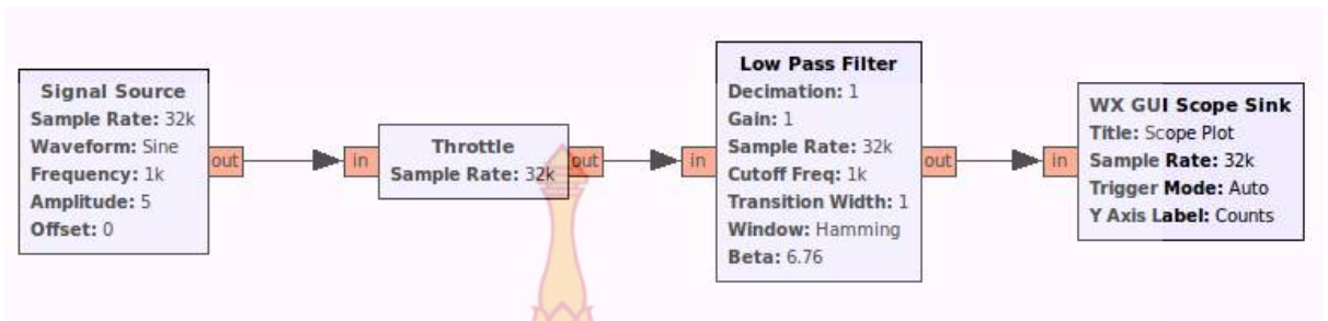
ภาพที่ 3-6 การทดลองวงจรกรองผ่านต่ำ
