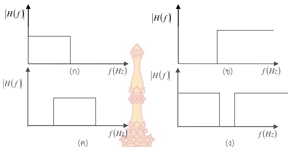
ภาพที่ 2-3 ทราแนส์เฟอร์ฟังก์ชันของวงจรกรองความถี่แบบต่าง ๆ (ก) Low pass filter (ข) High pass filter (ค) Band pass filter (ง) Band reject filter
