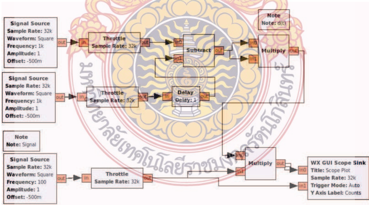
รูปที่ 6.1 การทดลองซิกซ์สัญญาณ
