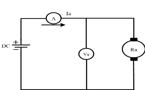
รูปที่ 5 วงจรถูกทดสอบความต้านทานอาร์เมเจอร์
