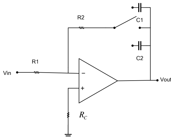
รูปที่ 3 ตัวควบคุมพีไอที่ใช้
