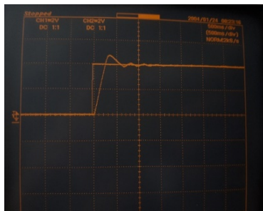
รูปที่ 11 ผลตอบสนองของระบบเมื่ออินพุตเป็นฟังก์ชันขั้นบันได
