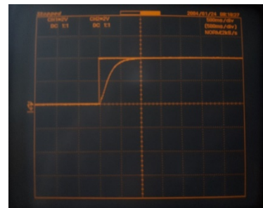
รูปที่ 11 ผลตอบสนองของระบบเมื่ออินพุตเป็นฟังก์ชันขั้นบันได
